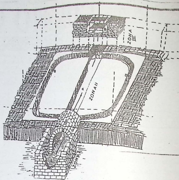
Figura 1. Croquis de un sistema de gloria simple.
